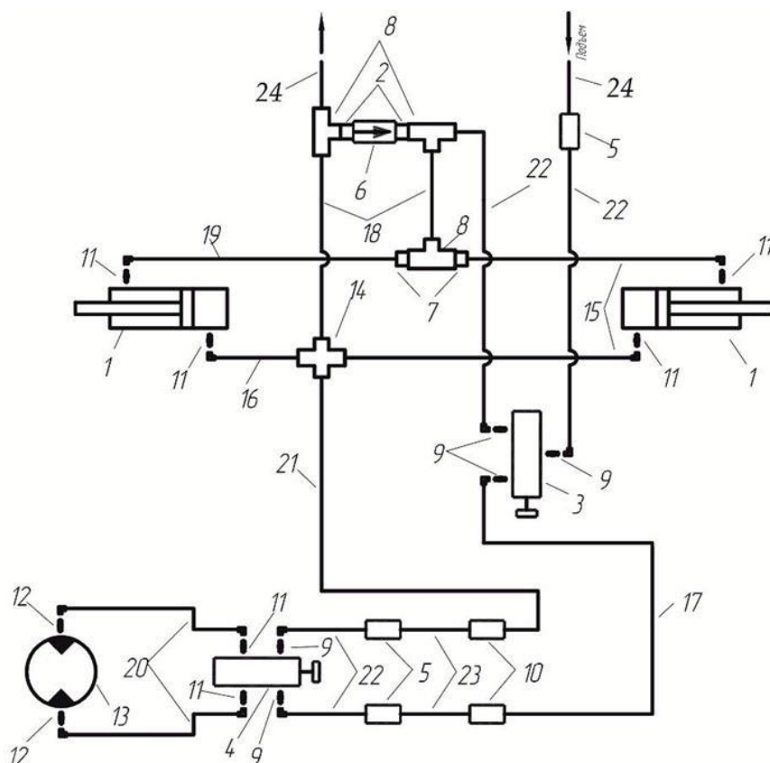
Рис.4.6.4 Компоненты гидросистемы управления «шнек – подъем/опускание крыльев» ПК-8.5, ПК-9.7 Компоненты гидросистемы управления «шнек – подъем/опускание крыльев» ПК-8.5, ПК-9.7
