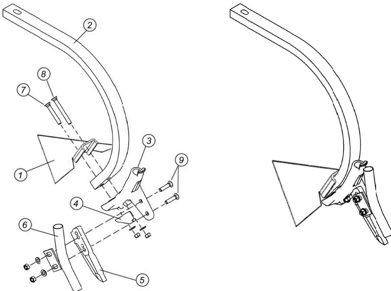
Рис. 4.5.4. Крепление сошников для ПК с раздельным высевом семян и удобрений
