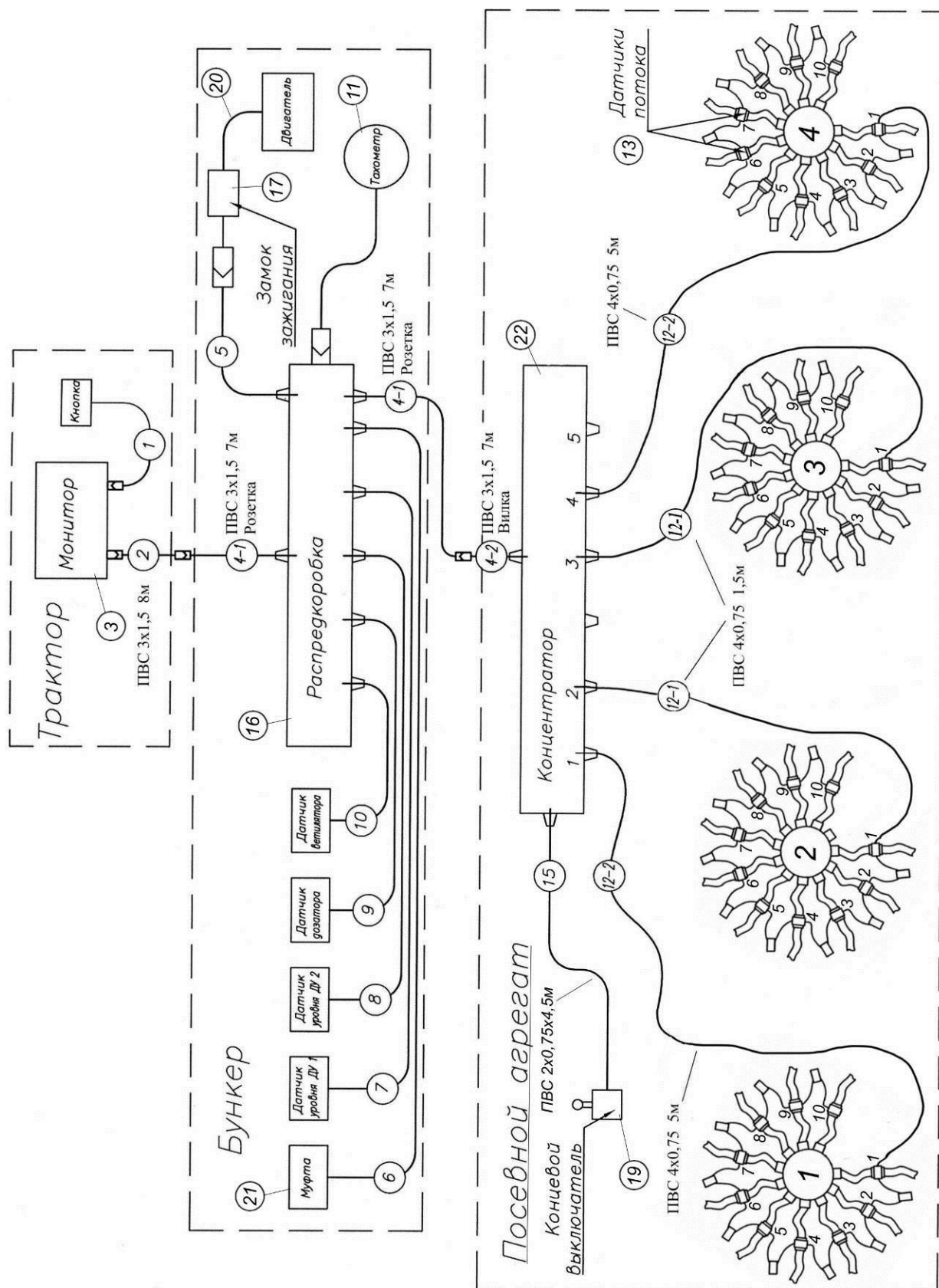
Схема электрическая соединений для ПК-12,2 "Кузбасс" с системой контроля засорения (бункер одноосный) Схема для ПК-8,5 отличается только количеством датчиков засорения (28шт.), для ПК-9,7 - (32 шт.).
