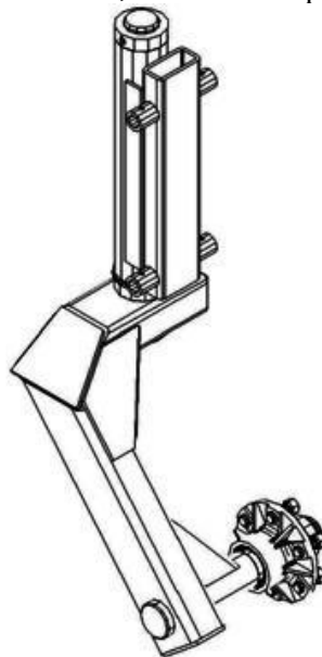
Рис. 4.4.2. Узел жёсткого одинарного колеса
