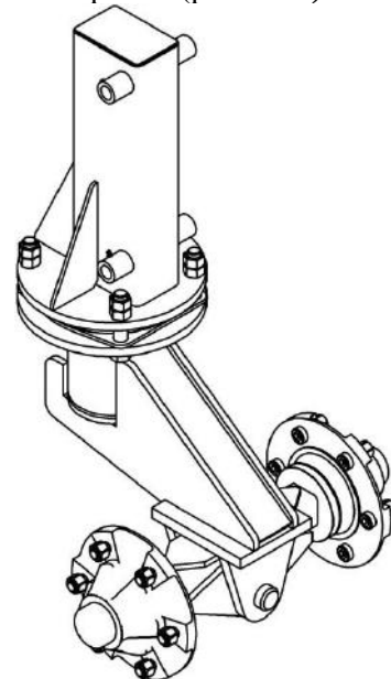
Рис. 4.4.3. Узел жёсткого двойного колеса нового образца
