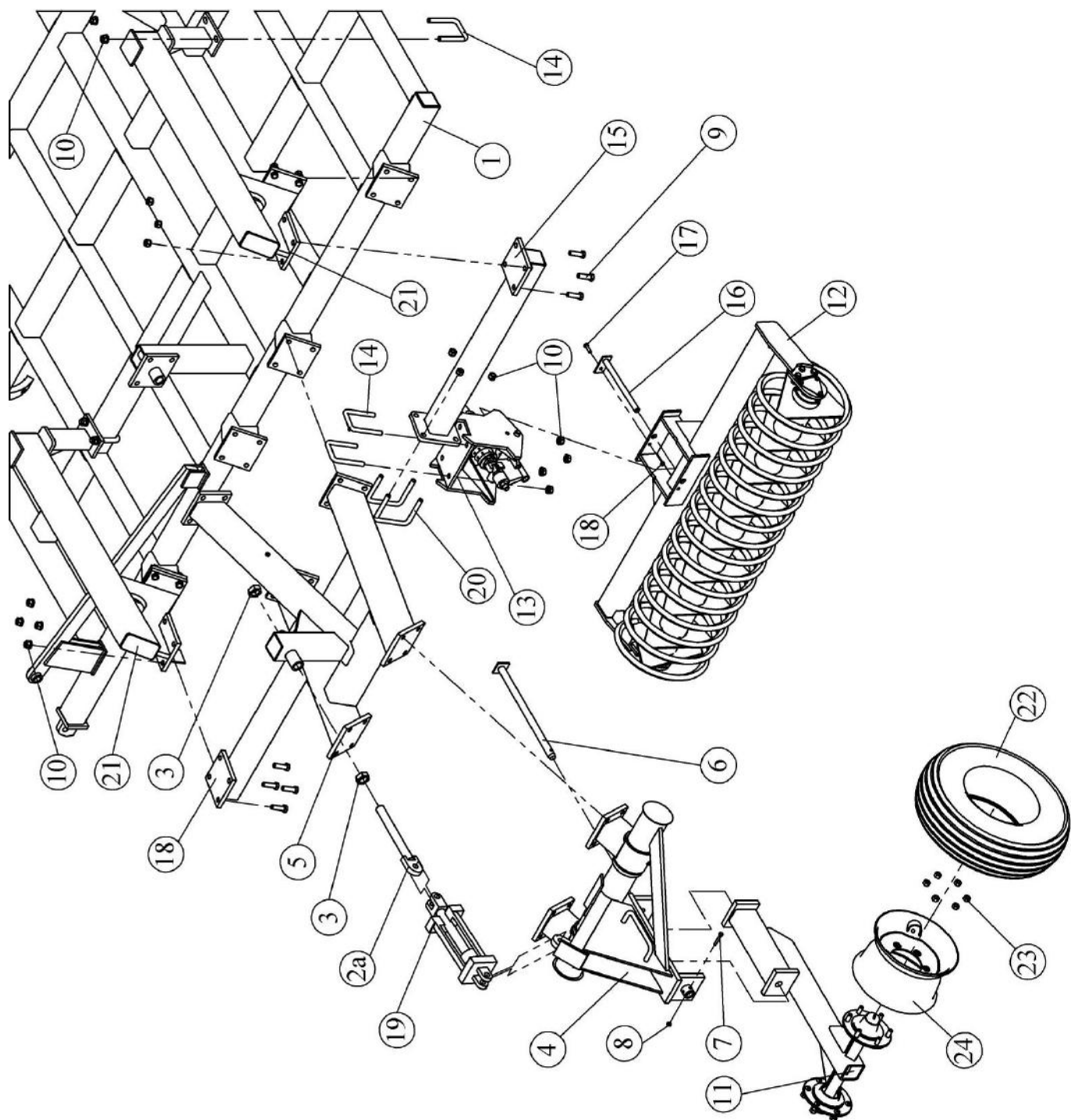
Рис. 7.1.2.2. Боковая рама, вставки с поворотным валом для ПК-12,2К.
